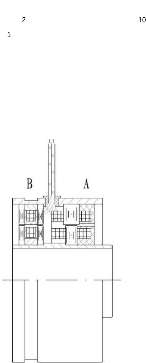
图 1、环形变压器式旋变结构示意图
